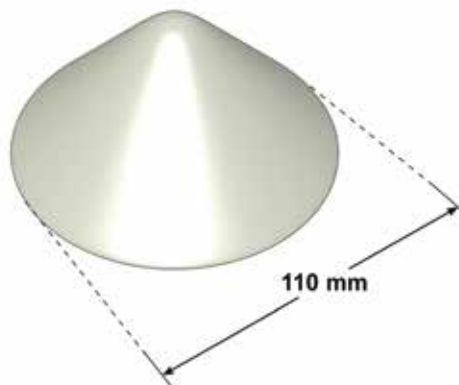
Tipo B: MAPEPLAN® T ANGOLO INTERNO CONICO PLUS Type B: MAPEPLAN® T INTERNAL CONIC CORNER PLUS
