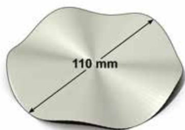
Tipo A: MAPEPLAN® T ANGOLO ESTERNO AD ONDA PLUS Type A: MAPEPLAN® T EXTERNAL WAVY CORNER PLUS
